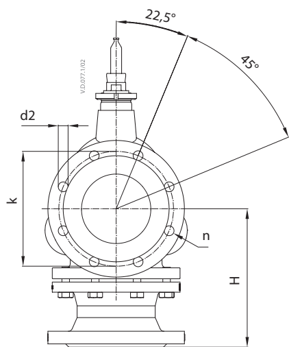
VF 3 DN 125-150
